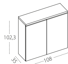
Elemento laterale 2 ante L cm 108
