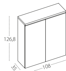
Elemento laterale 2 ante L cm 108
