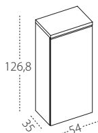
Elemento laterale 1 anta L cm 54
