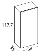
Pensile 1 anta L cm 54
