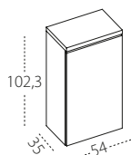
Elemento laterale 1 anta L cm 54
