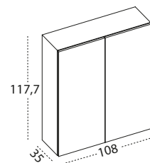
Pensile 2 ante L cm 108
